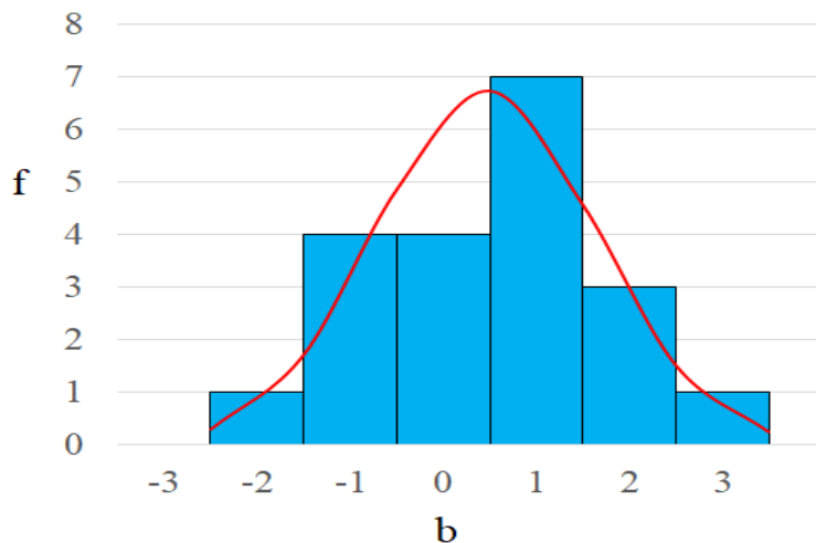
1-rasm. Rash modeli bo'yicha hisoblangan test topshiriqlari qiyinlik darajalari taqsimotini (ustunlar) normal taqsimot (uzluksiz chiziq) bilan taqqoslash
