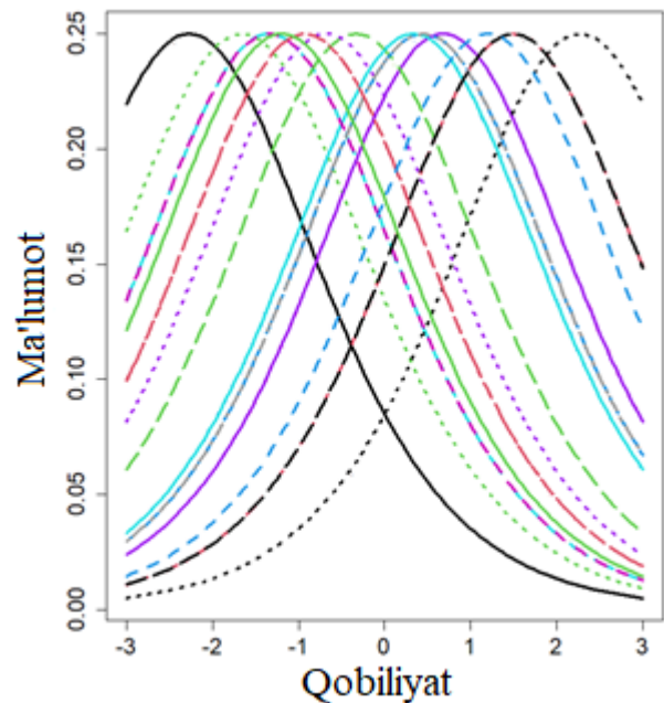
3-rasm. Element ma'lumoti chiziqlari
