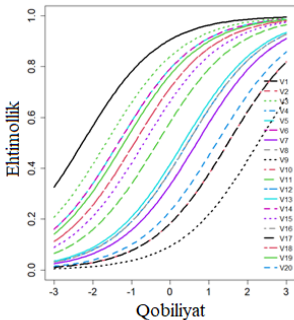
2-rasm. Element tavsifi chiziqlari
