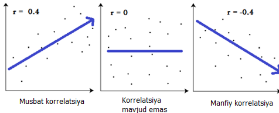
1-rasm. Pirson korrelatsiya koeffitsiyenti grafigi
