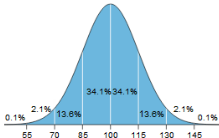
1-rasm: IQ testlarida ishlatiladigan normal taqsimot.
